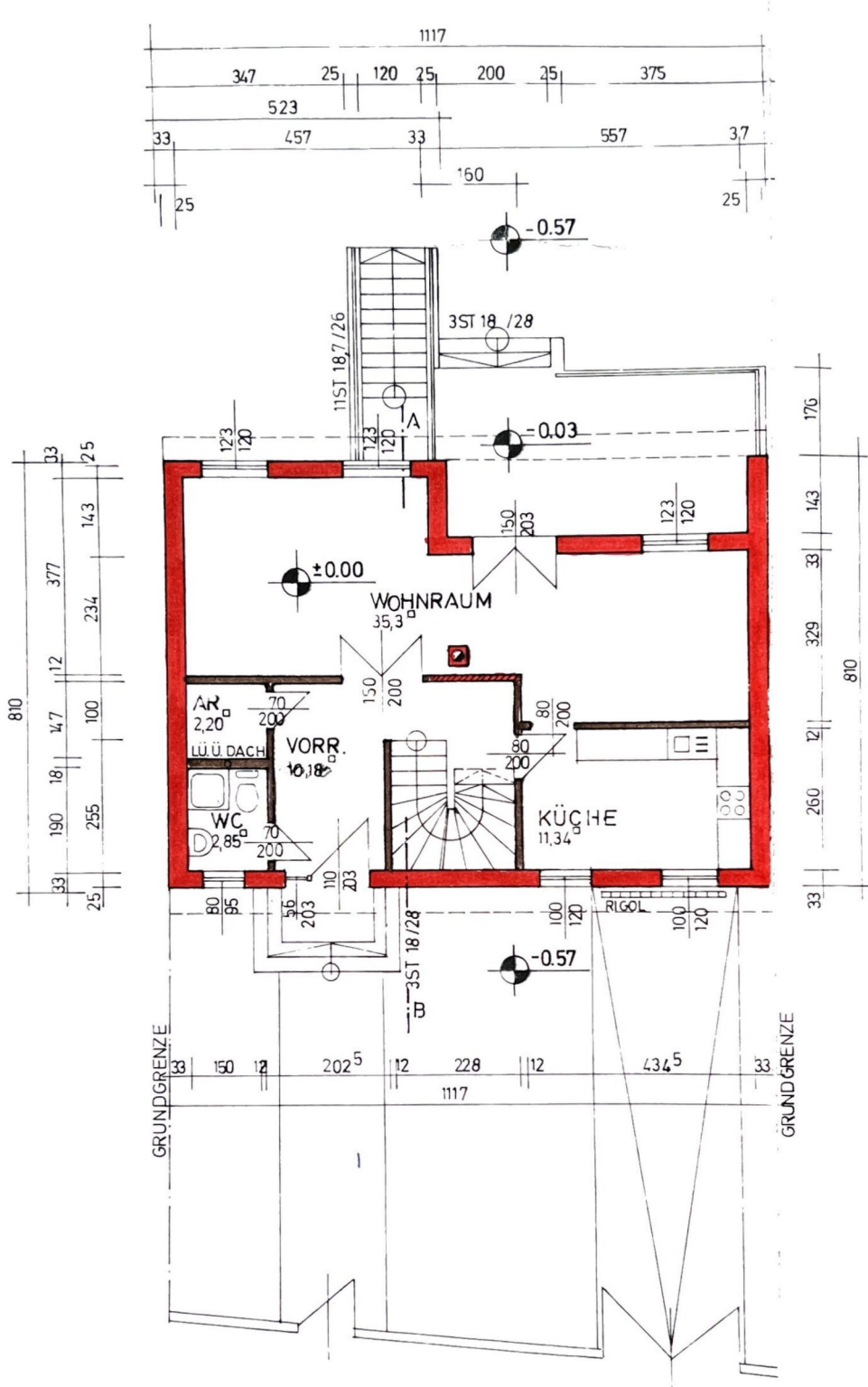
ERDGESCHOSS WOHNNUTZFLÄCHE 61,87 m 2
